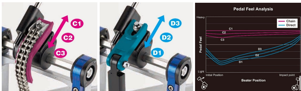
ダブルチェーンドライブ（左）とダイレクトドライブ（右） それぞれでの調整イメージ
