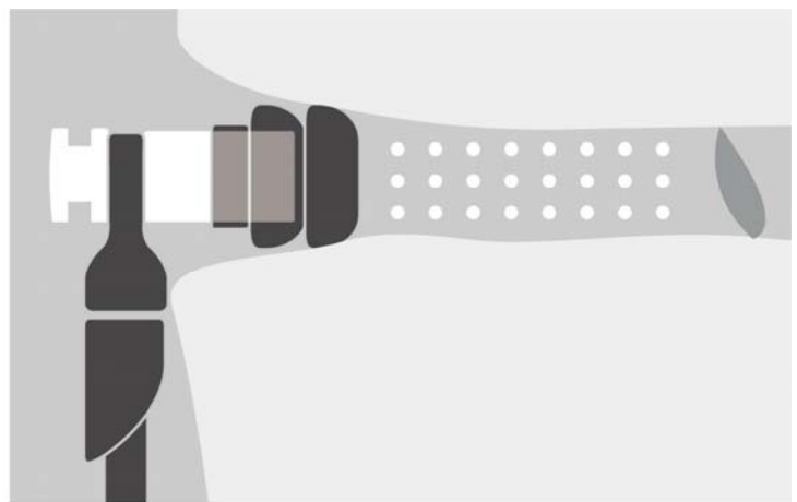
外耳道内の不要反射を低減する設計
