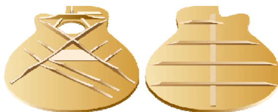
(左) 表板の新スキャロップブレッシング / (右) 裏板のカッタウェイ専用ブレッシング
